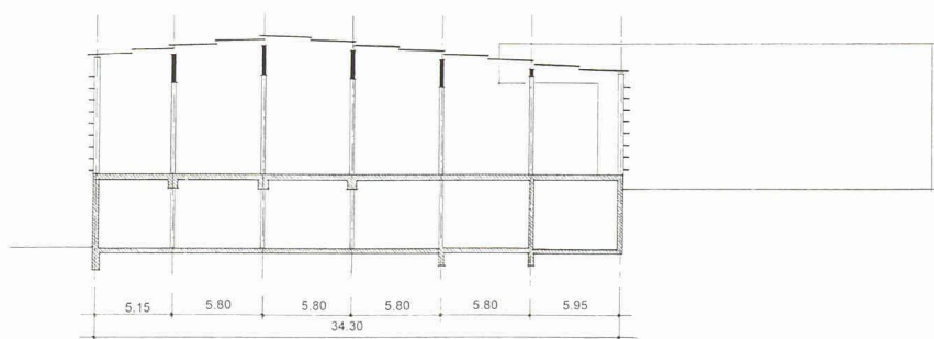
Längsschnitt
