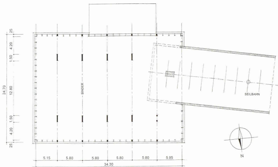
Grundriss Halle
